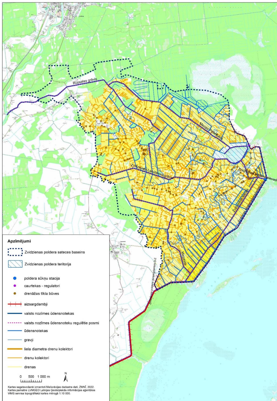
1.4.attēls. Zvidzienas poldera teritorija un būves. (Avots: Balstoties uz ZMŅI informācijas.)
